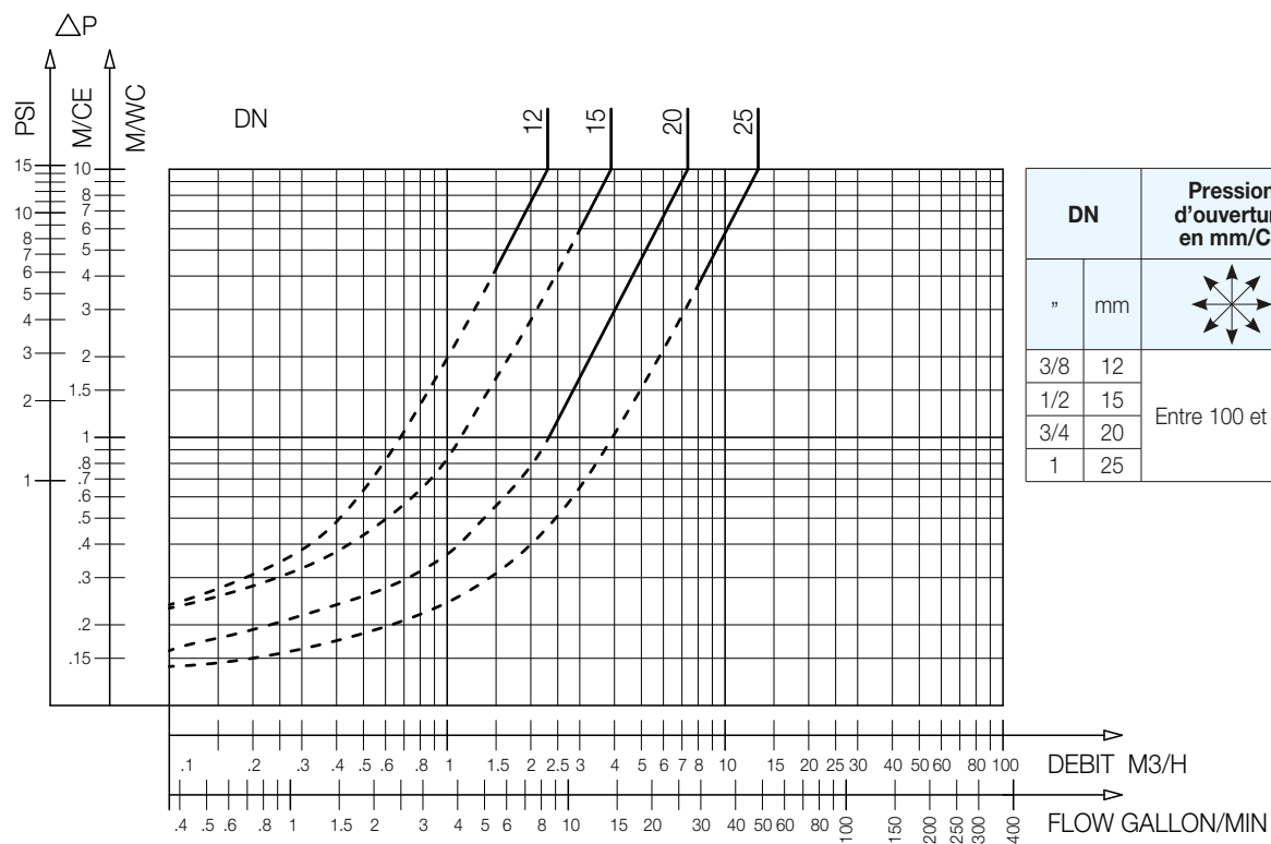
290 D - Abaque des pertes de charge
