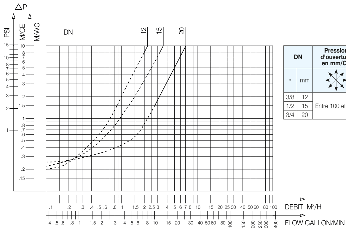
290 P - Abaque des pertes de charge
