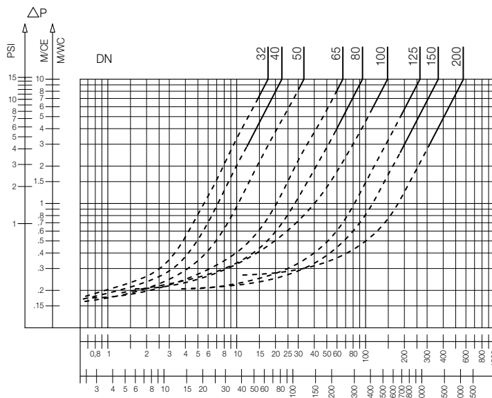
802 - Abaque des pertes de charge
